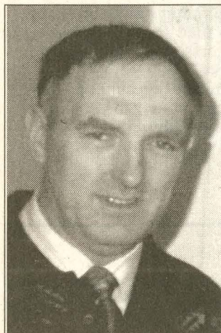
Aage G. Folkmann
